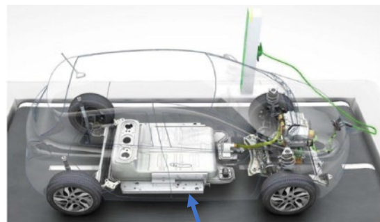
Pack batterie
